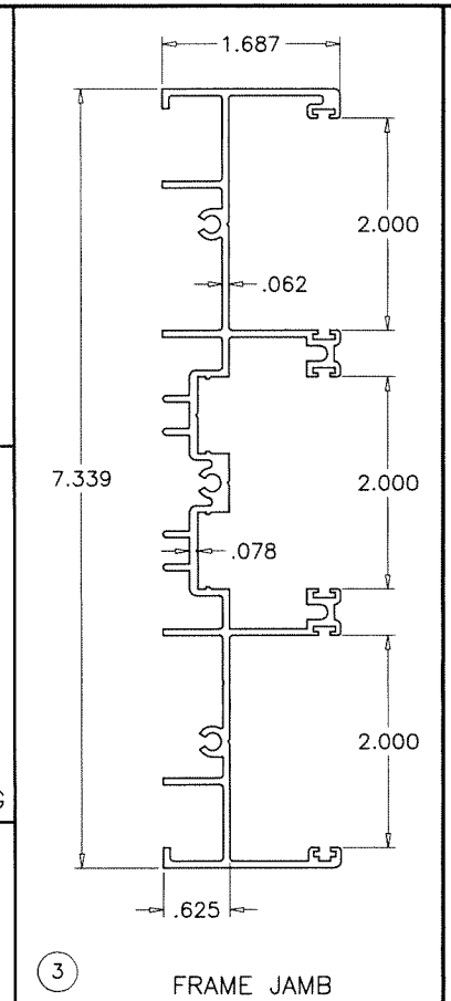
FRAME JAMB
